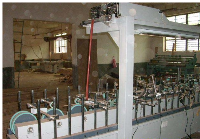
线条包覆机
